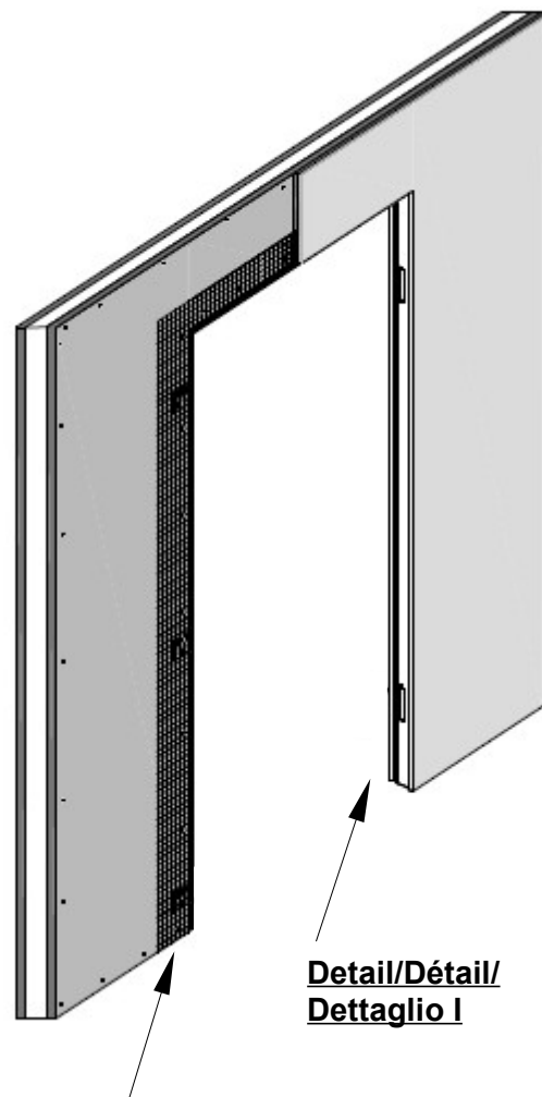
Detail/Détail/Dettaglio K
