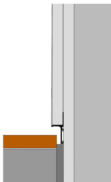
Drywall construction
